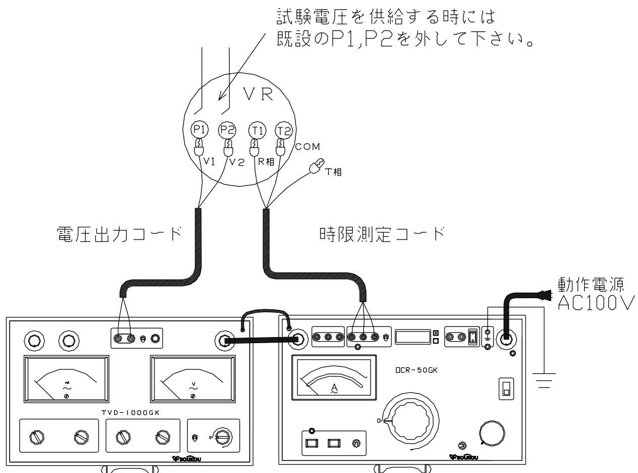
図4：試験回路図（停電状態）
