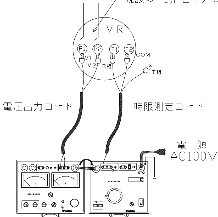
図18：試験回路図(停電状態)
