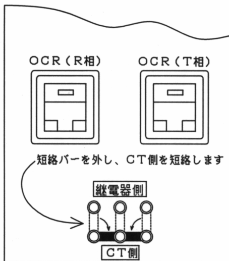
図2：試験用端子の短絡方法
