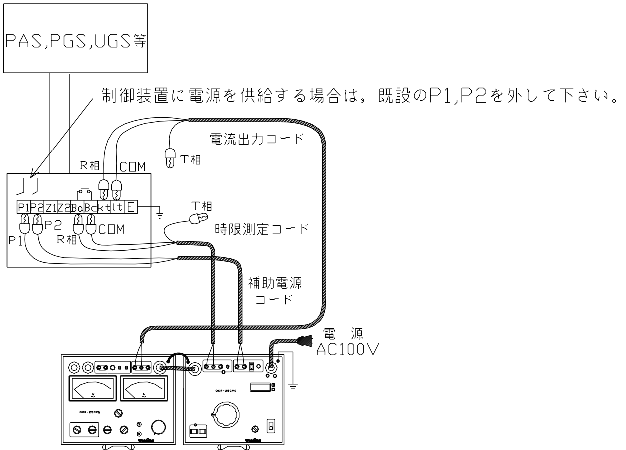
図15：試験回路図—PAS, PGS等の単体試験（停電状態）
