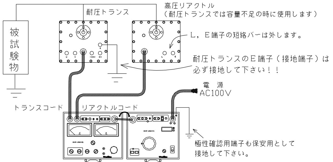
図19：試験回路図
