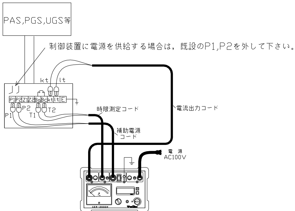
図4：試験回路図－PAS,PGS等の単体試験（停電状態）
