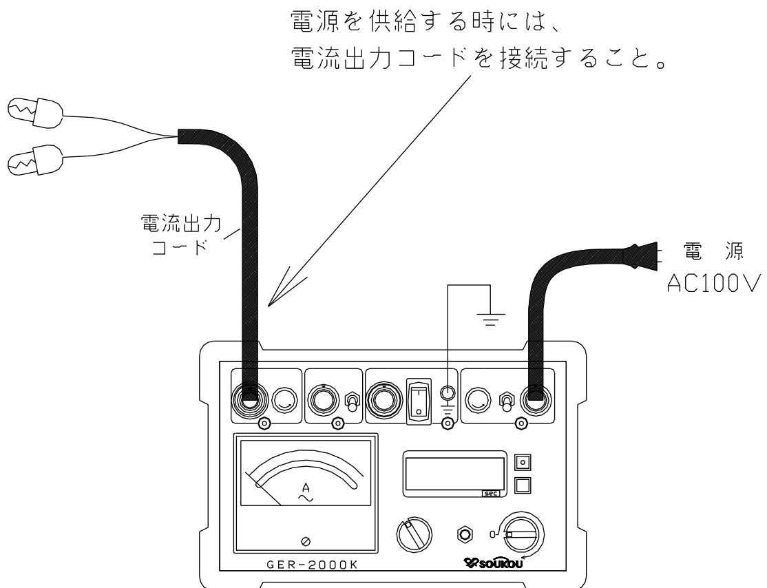
図1：電源の供給
