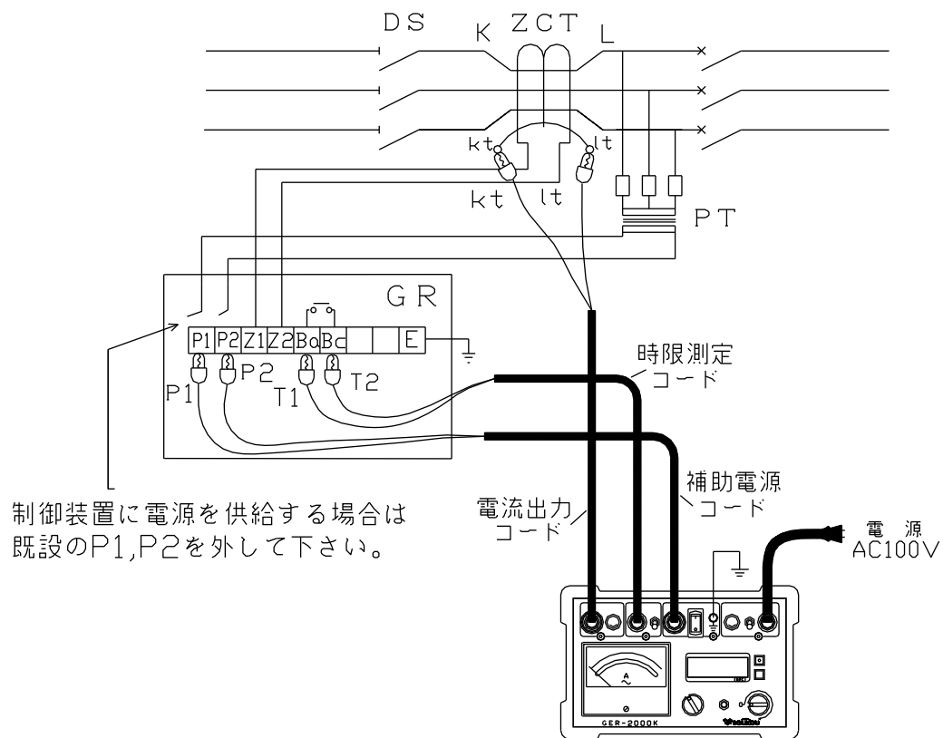
図3：試験回路図
