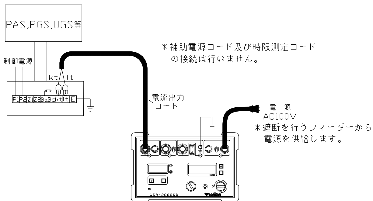
図5：試験回路図ーPAS,PGS等の連動試験（受電状態）
