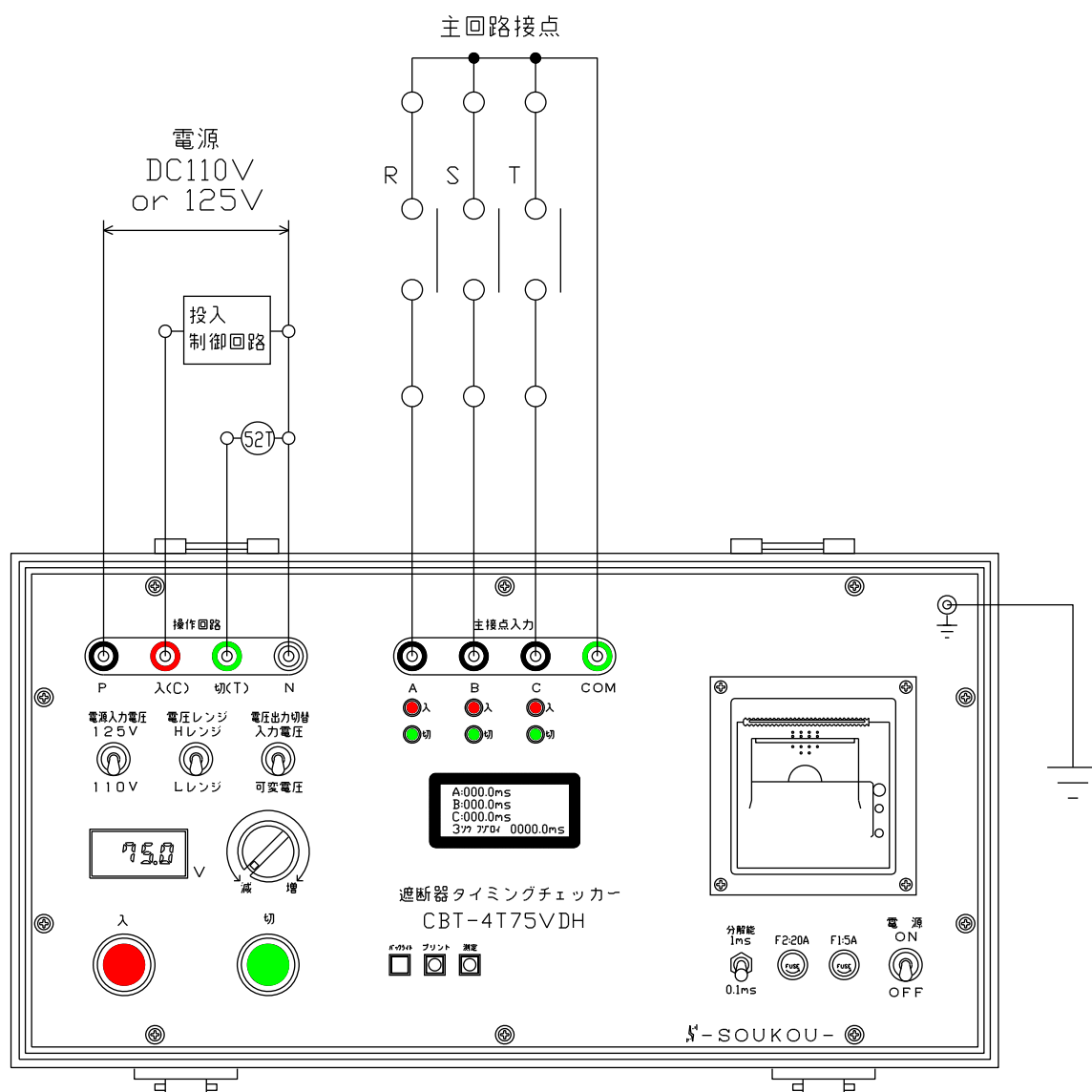
図1：接続例
