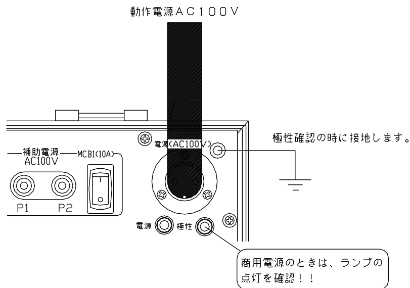
図4：電源の極性確認方法
