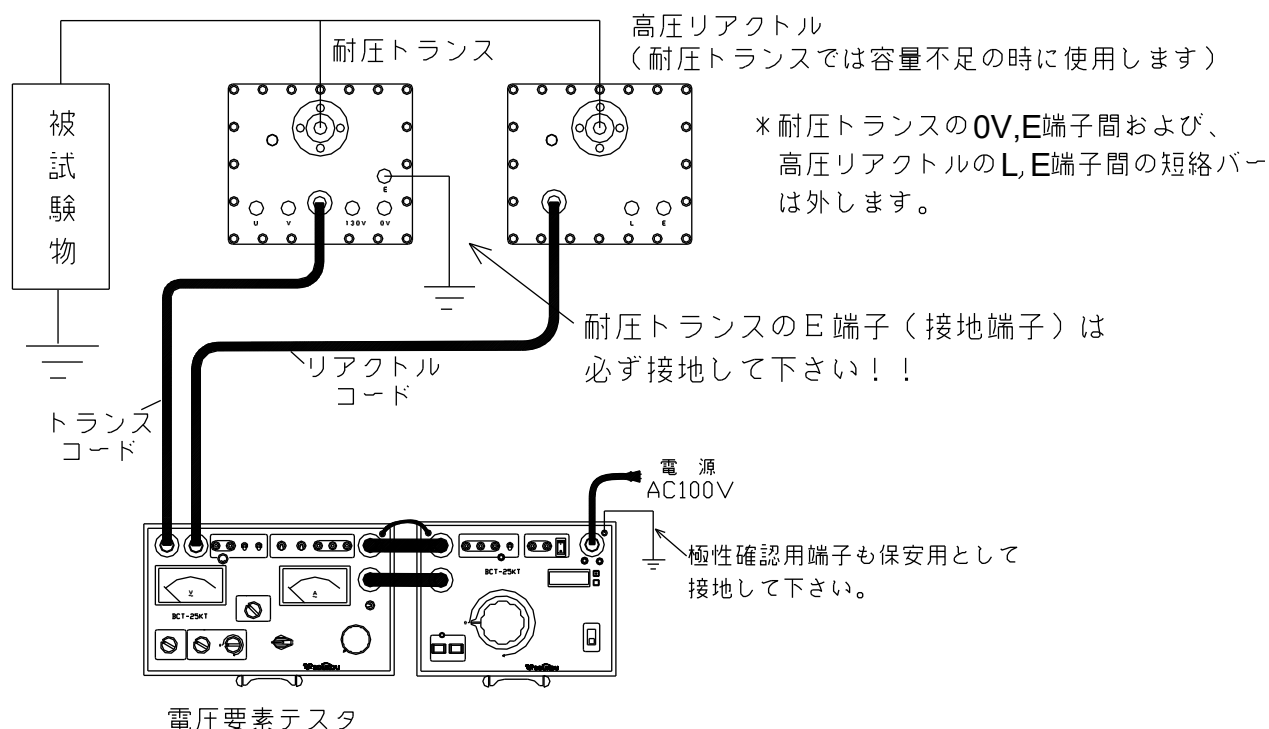
図20：試験回路図
