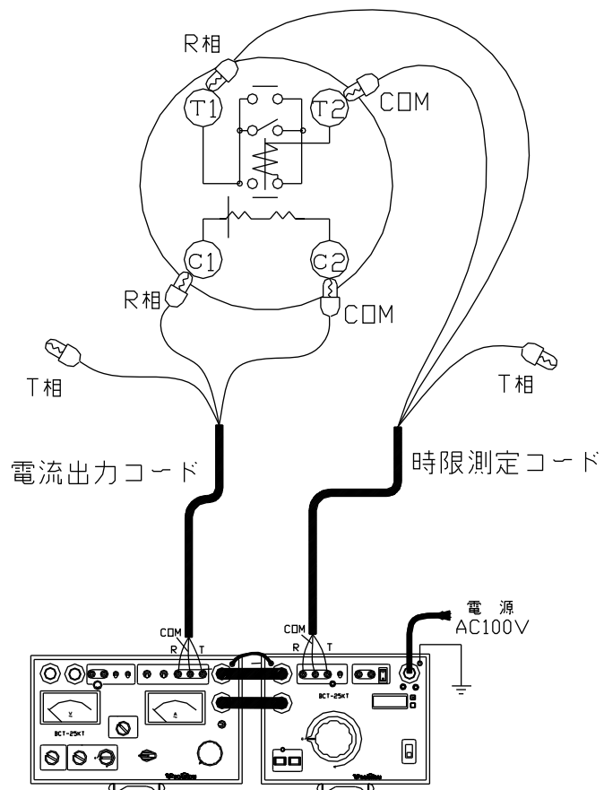
図7：試験回路図－R相単体試験（無電圧引き外し方式）
