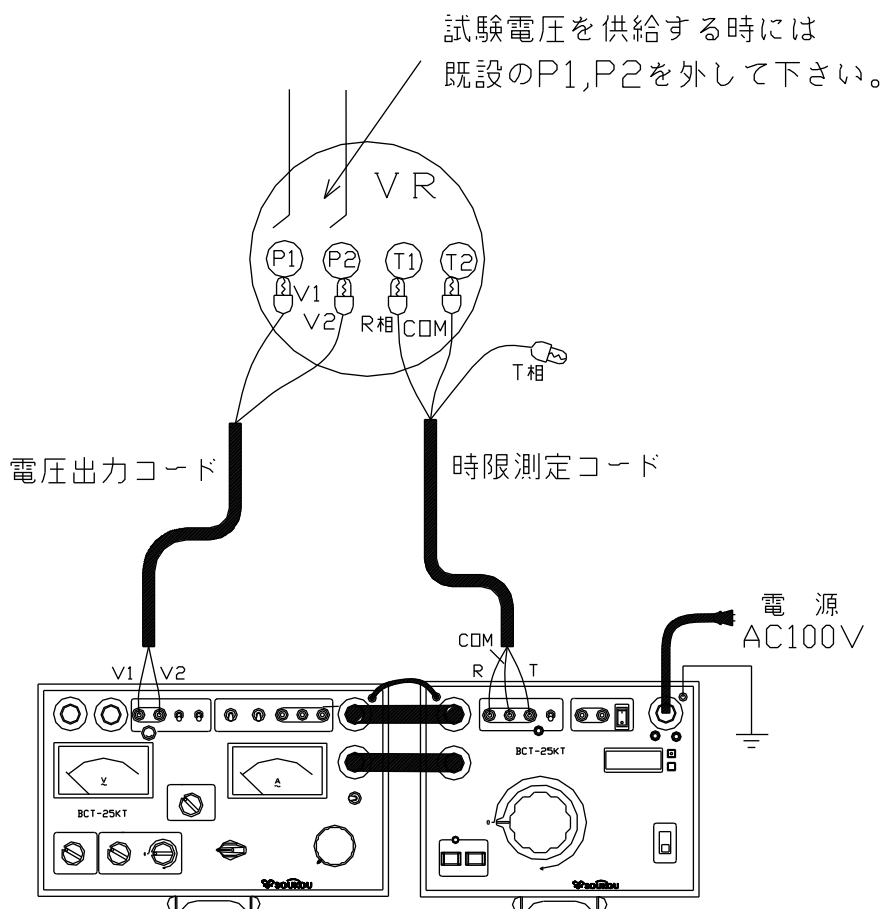
図19：試験回路図(停電状態)
