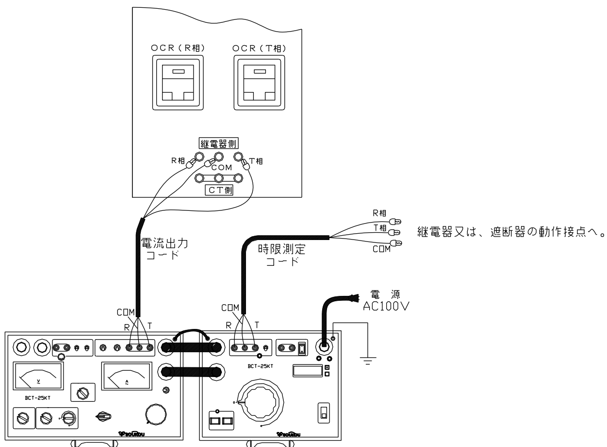
図5：試験回路図（構成）
