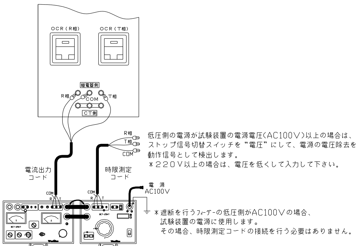
図9：試験回路図一連動試験（受電状態）
