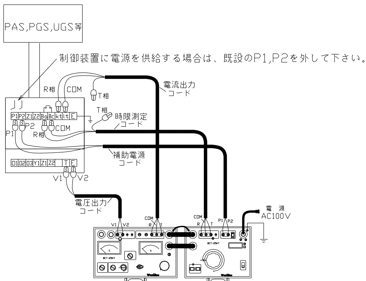
図17：試験回路図－柱上の単体試験（停電状態）
