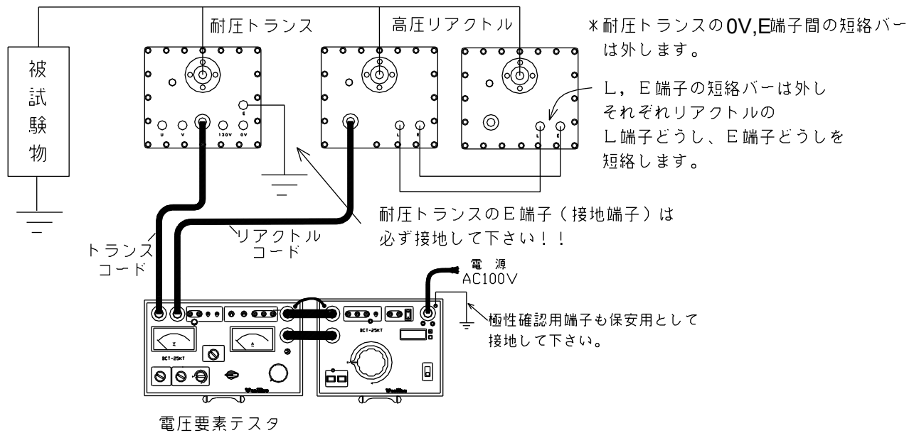
図22：リアクトルを複数使用する場合
