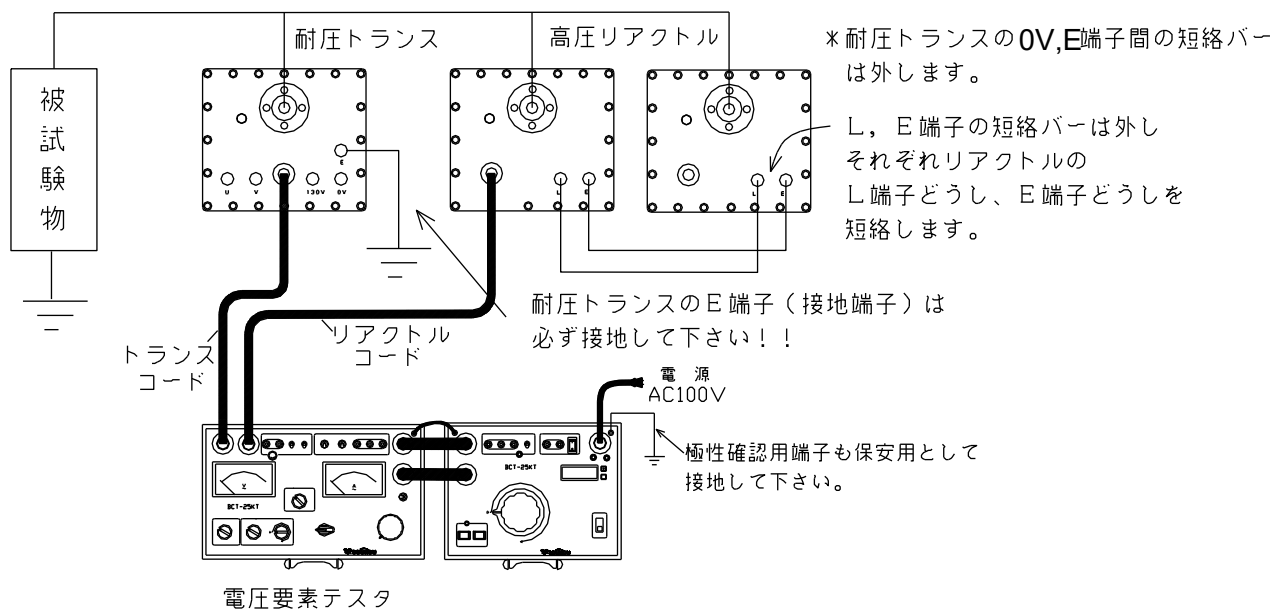
図21：試験回路図
