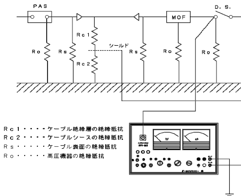
図5：PAS,MOF を切りはなさずケーブル単体の絶縁抵抗を測定する（ガード接地方式）
