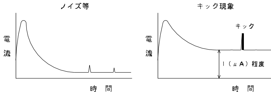
図8：キック現象の例
