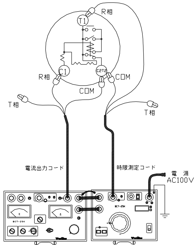
図6：試験回路図一R相単体試験（2次電流引き外し方式）
