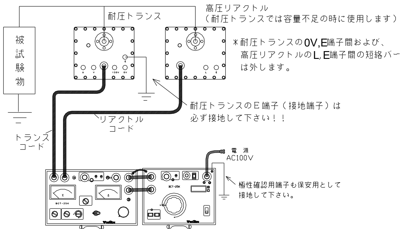
図21：試験回路図
