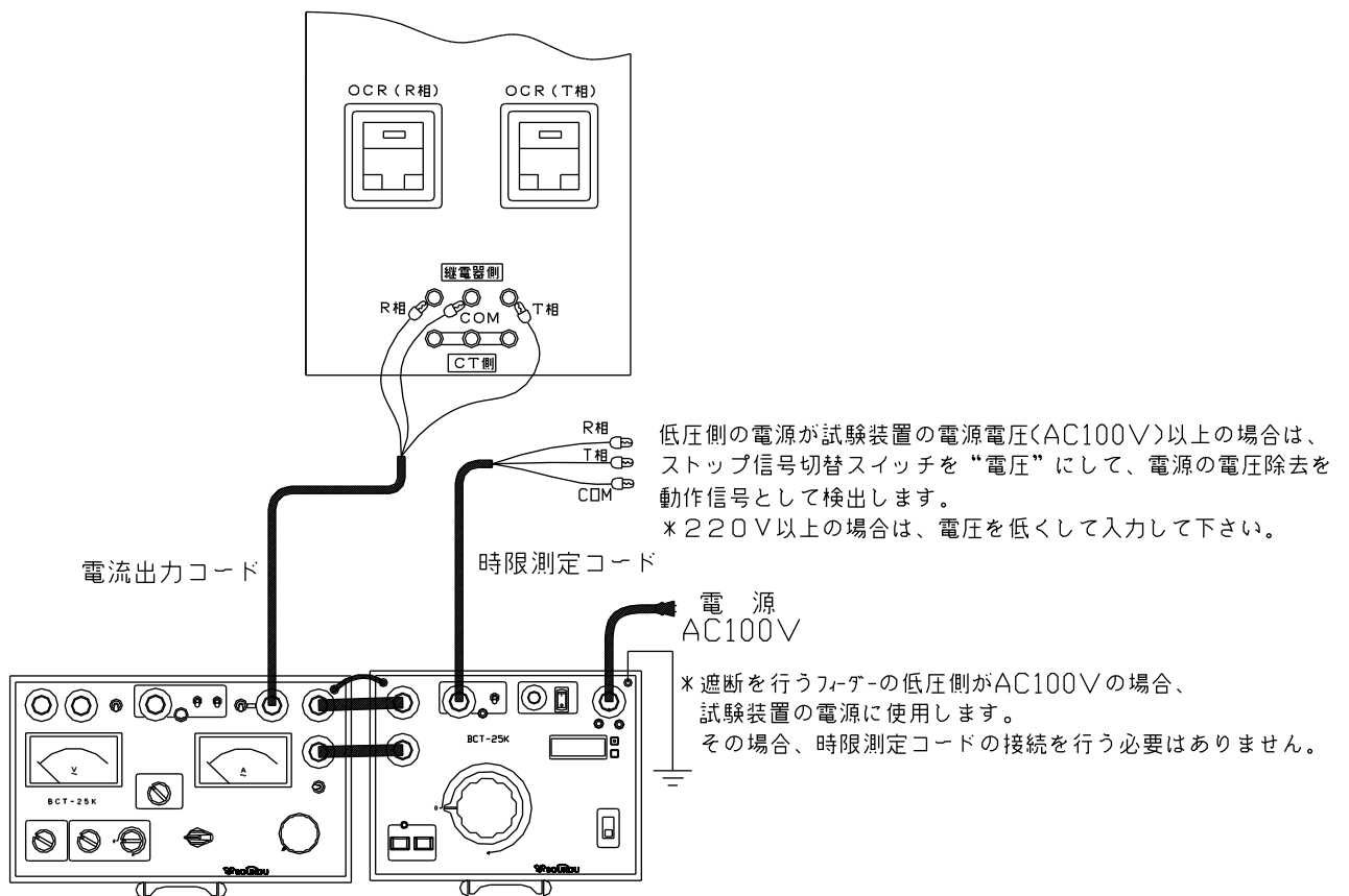
図9：試験回路図一連動試験（受電状態）
