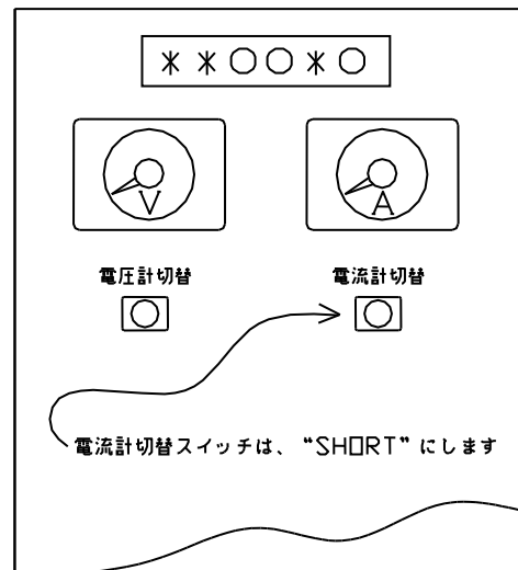
図3：電流計切替スイッチの位置
