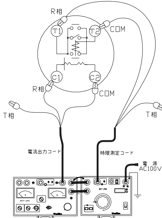
図7：試験回路図一R相単体試験（無電圧引き外し方式）
