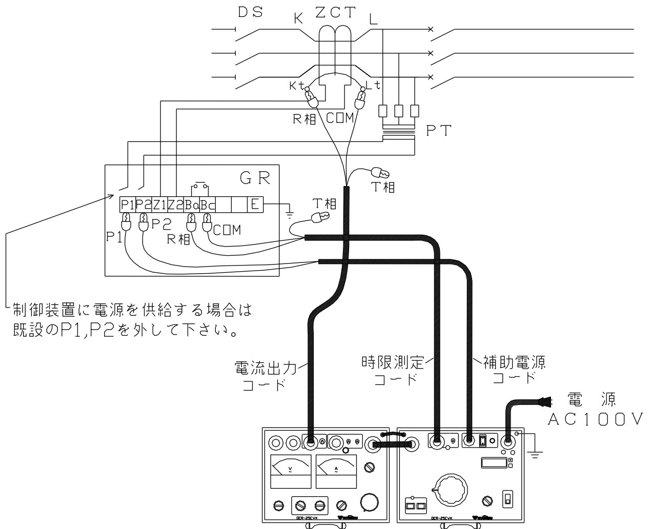
図14：試験回路図一電気室の単体試験（停電状態）
