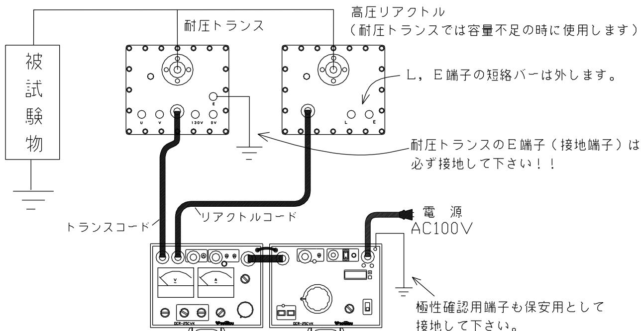
図20：試験回路図
